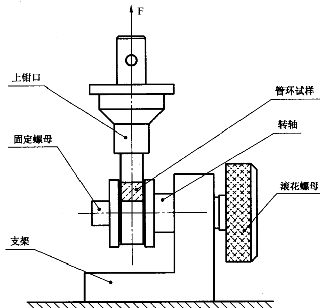
图 A.1 管环转盘支架示意图
