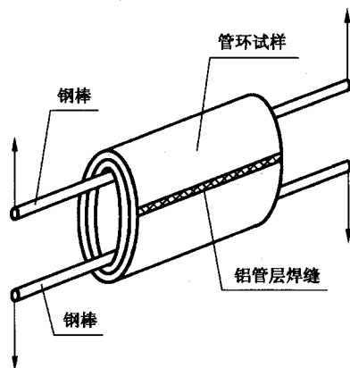
图 2 管环径向拉力试验
